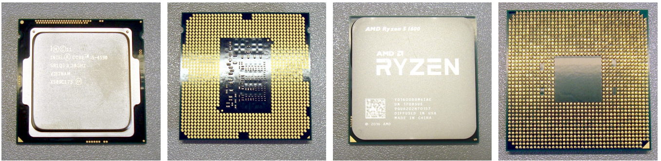
Intel CPU Oberseite Intel CPU Unterseite AMD CPU Oberseite AMD CPU Unterseite
